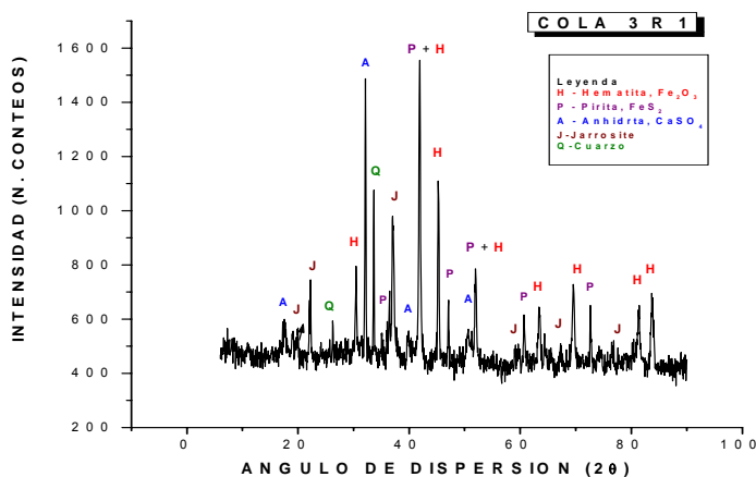
Figura 5 Difractograma del residuo del proceso HPAL de nódulos de Mn ( P-7)
