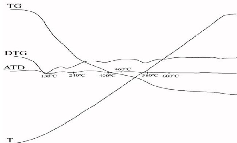
Figura 4 Análisis Térmico de la muestra de nódulos de manganeso
