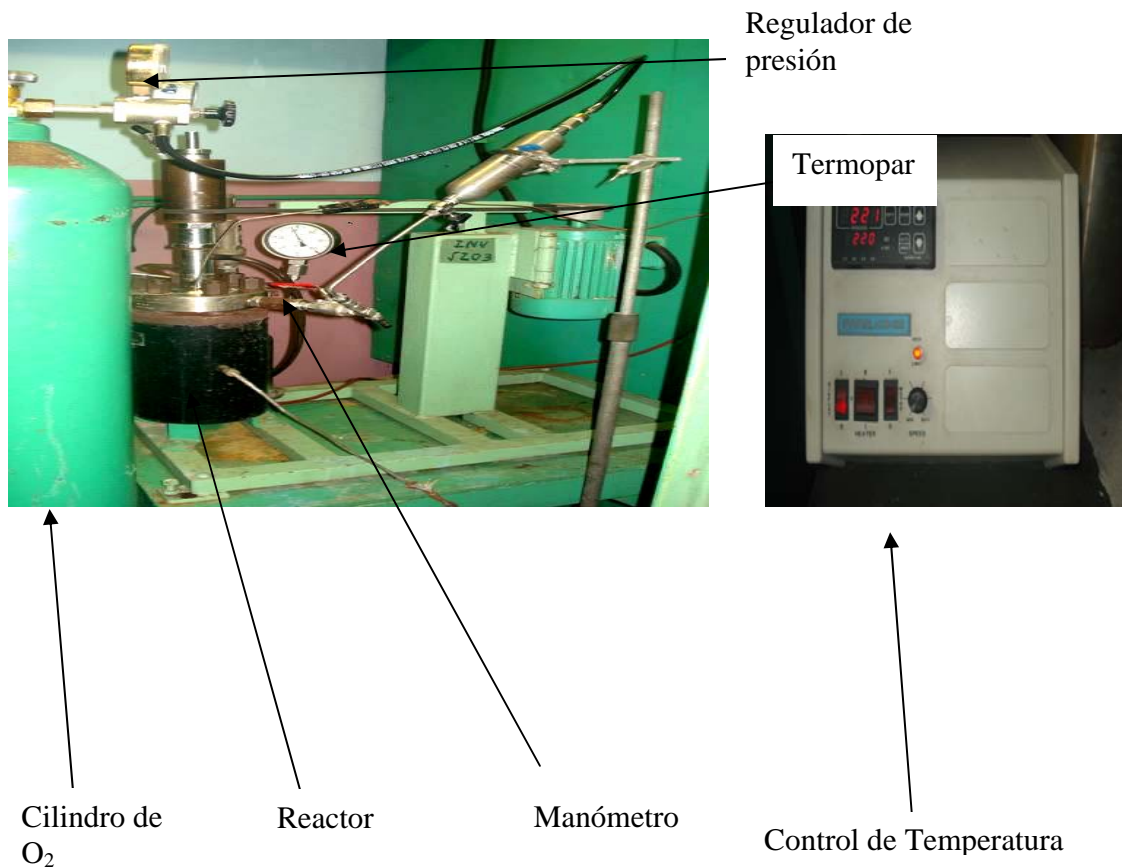
Figura 2 Equipamiento utilizado en el proceso de lixiviación.
